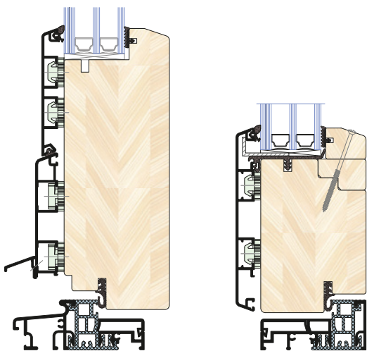
Doorsneden van deursystemen
