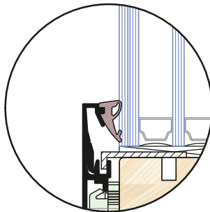
Optionele beglazing met aluminium beglazingsprofiel
