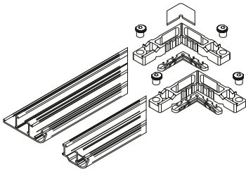
Onderdelen samengeperste hoeken
