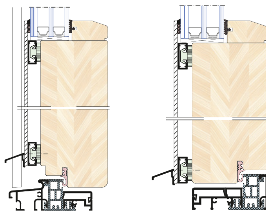
Doorsneden van paneeldeuren
